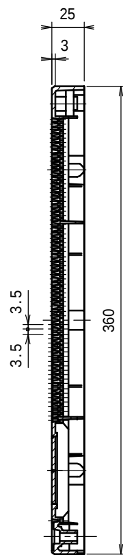
A-A断面図
